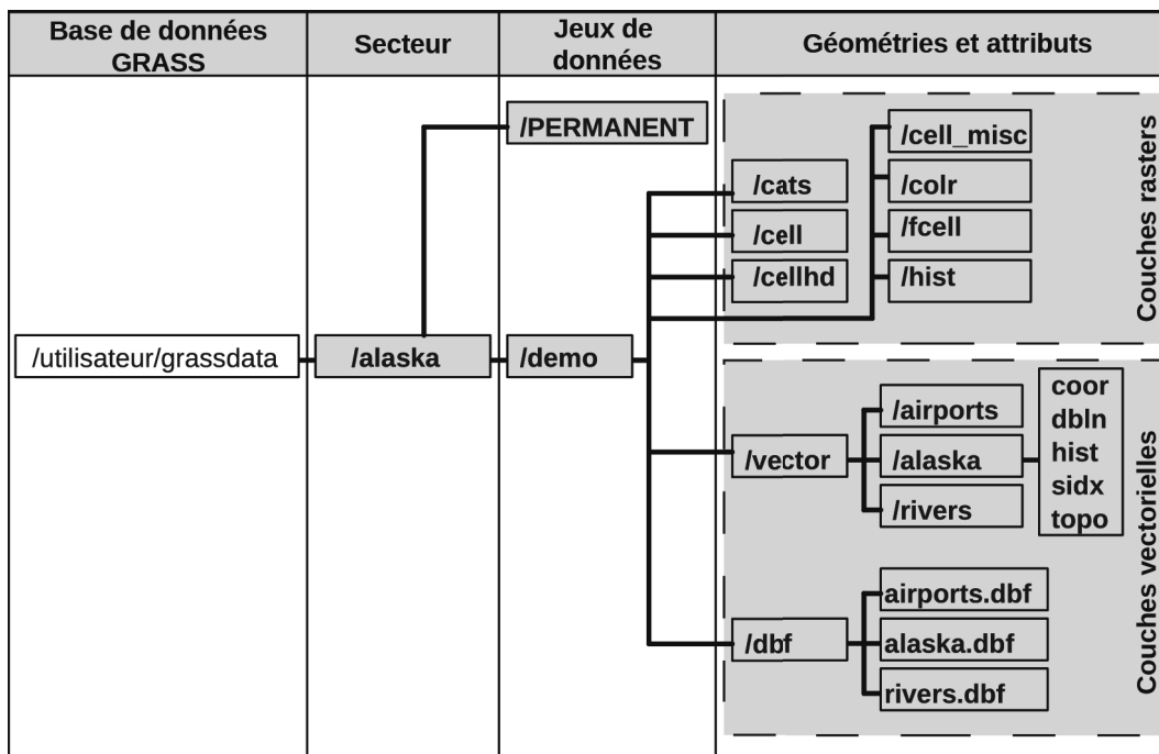
FIGURE 8.1.: Données GRASS dans le SECTEUR Alaska (adapté de Neteler & Mitasova 2008 [3])
