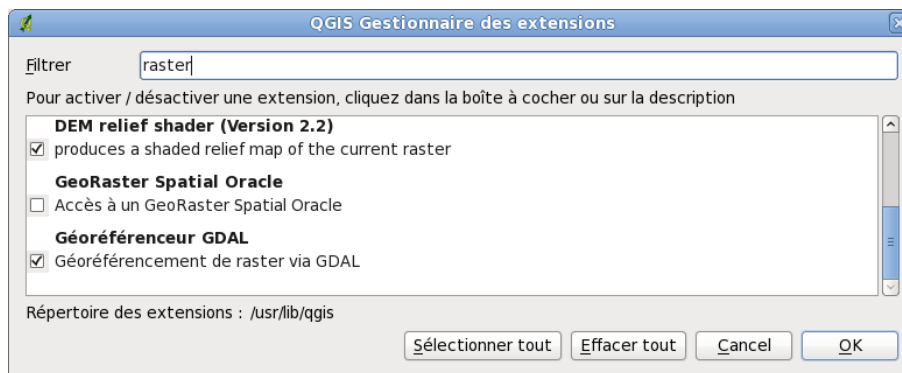
FIGURE 10.1.: Gestionnaire d'extension 🐧
